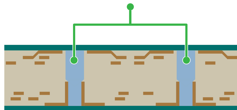
(多層基板 断面図)
